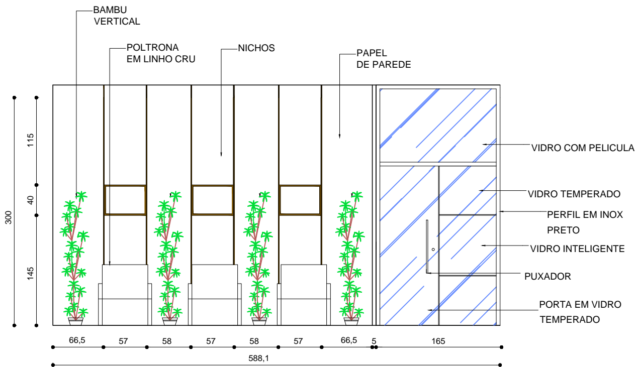
ELEVACAO A ESC.: 1/50
