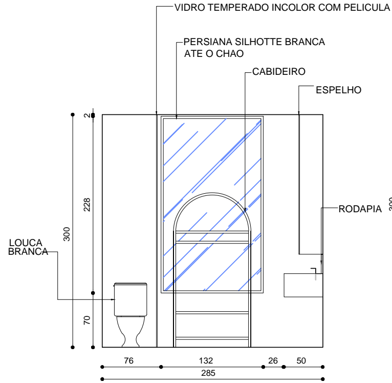
ELEVACAO D ESC.: 1/50
