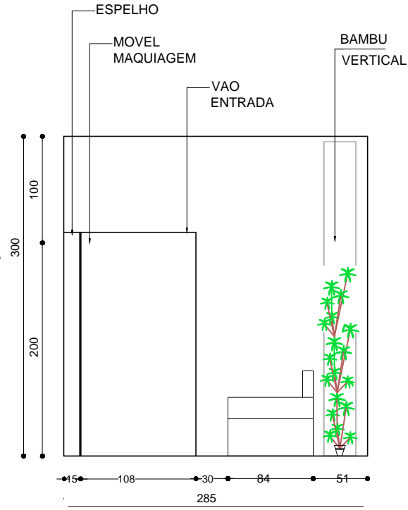
ELEVACAO C ESC.: 1/50
