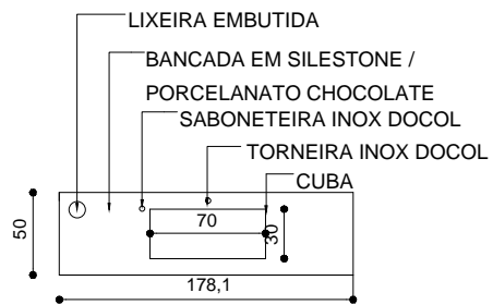
VISTA SUPERIOR BANCADA ESC.: 1/50
