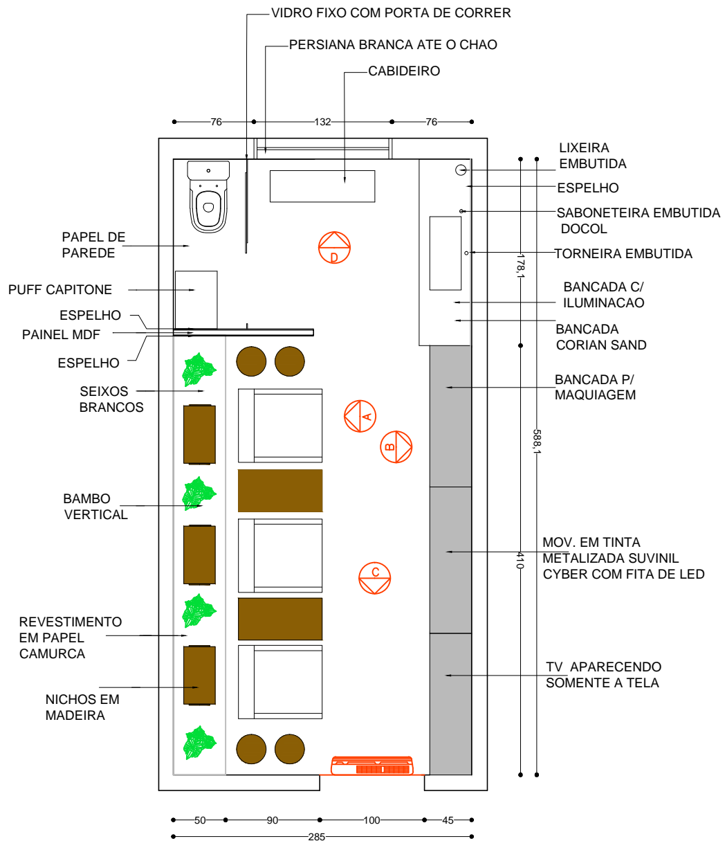
LAYOUT ESC.: 1/50
